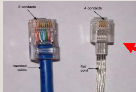
Phone Cable
